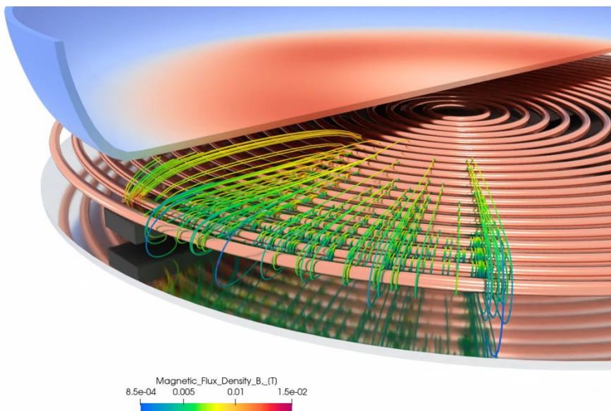
Auslegung eines Induktionskochfeldes: Die per Simulation optimierten Spulen gestatten eine präzisere Erwärmung und reduzierte Taktzeiten. (Quelle CENOS)
