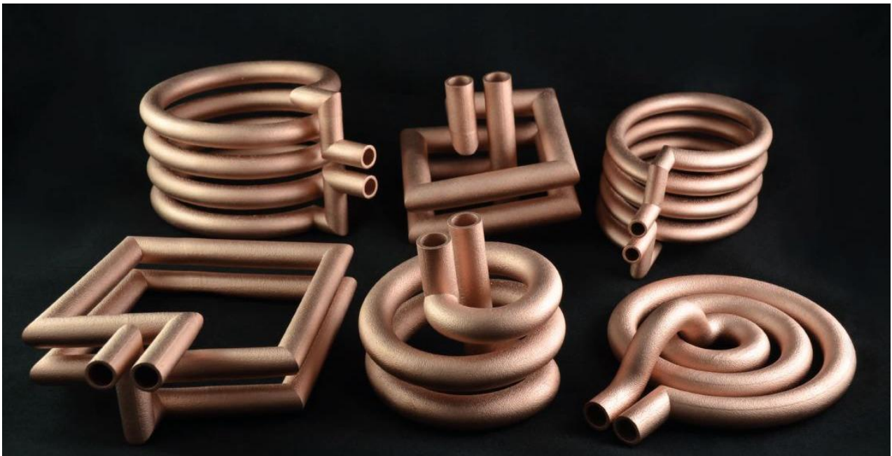
Der von ProtIQ entwickelte Prozess zur Verarbeitung von hochleitfähigem Reinkupfer im selektiven Laserschmelzprozess erlaubt die Herstellung innovativer Bauteile für die Elektroindustrie
